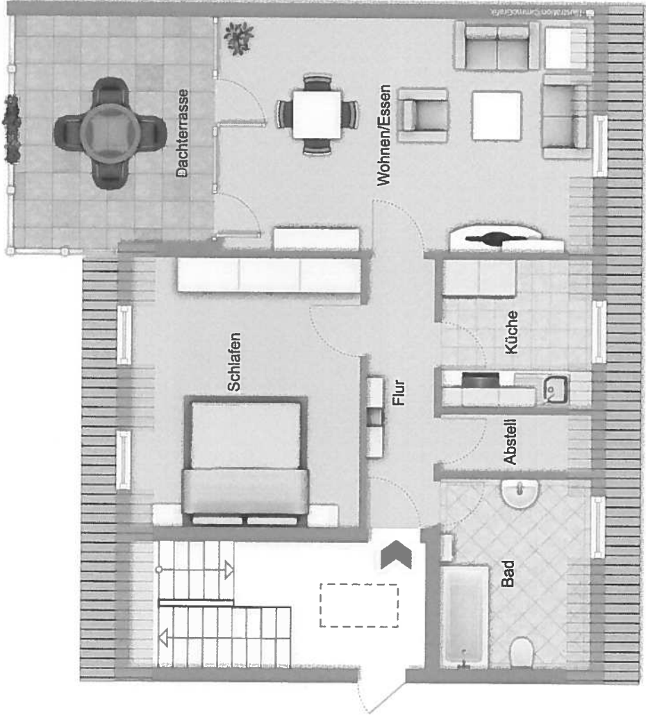
Grundriss
